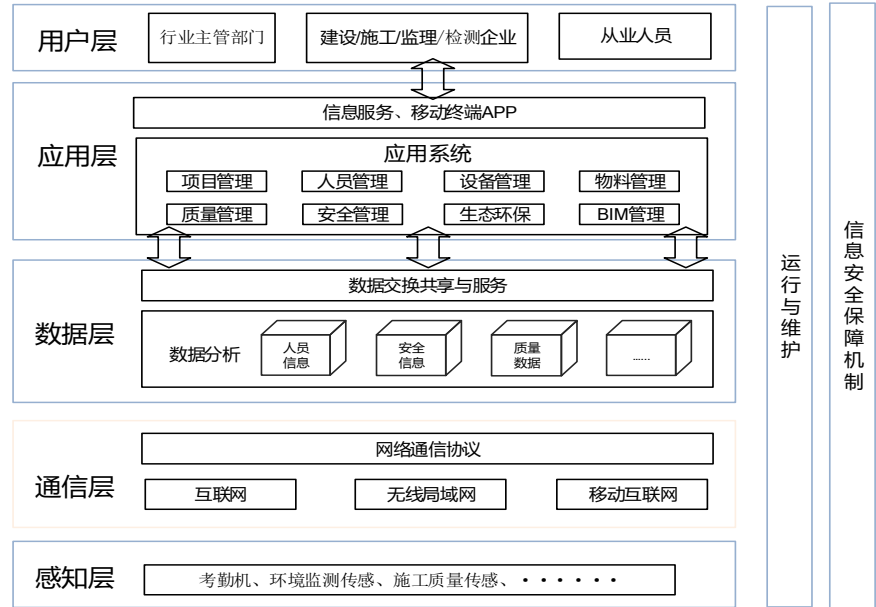
图1 智慧工地架构图
