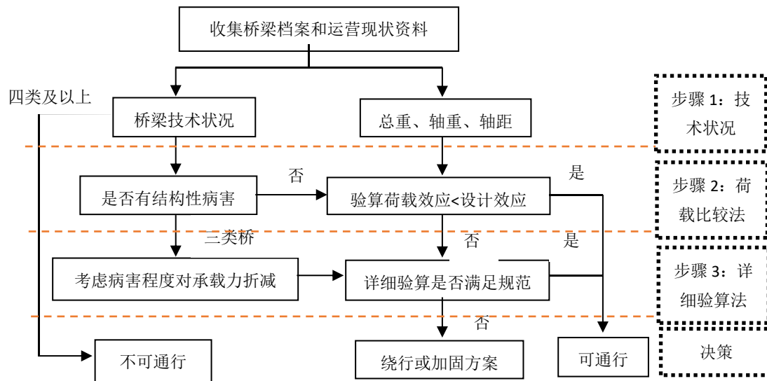
大件运输桥梁承载许可验算框图
