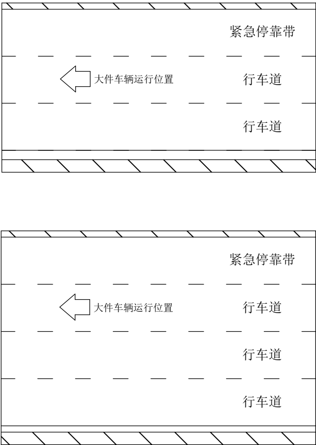
考虑实际运营情况的大件运输车辆横向布置位置示意
