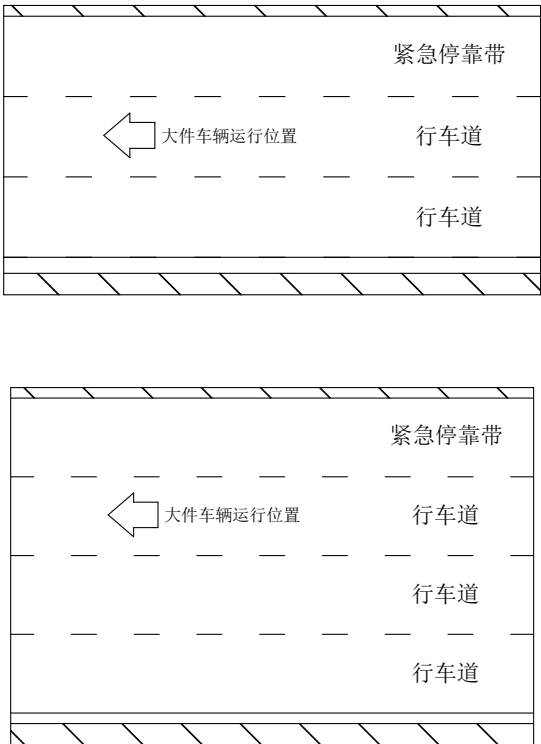
图 1 考虑实际运营情况的大件运输车辆横向布置位置示意
