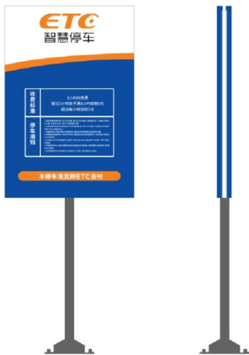
图 A.5 路内停车位停车立牌标识示意图
